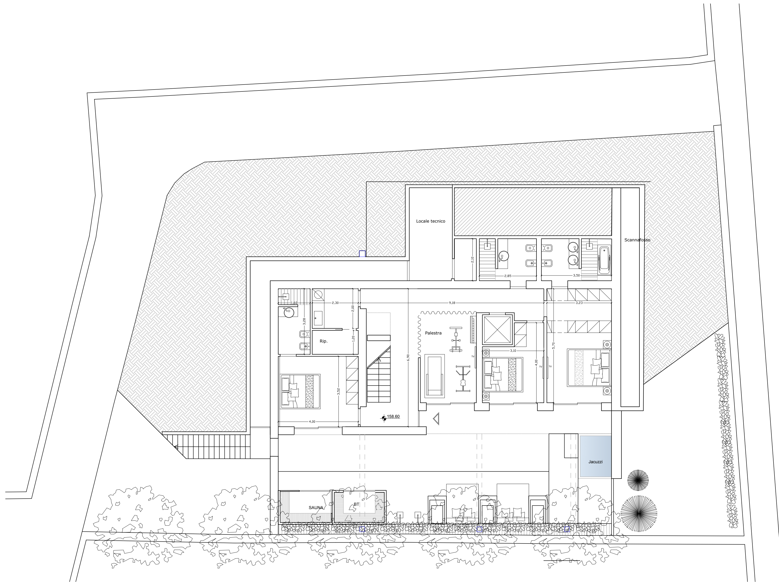
Planimetria piano interrato
